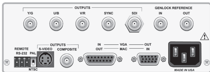
Scan Do Pro II および Pro II/D 背面パネル
